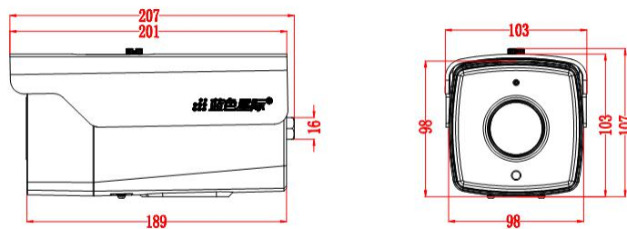
产品尺寸图
