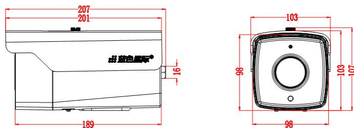
产品尺寸图
